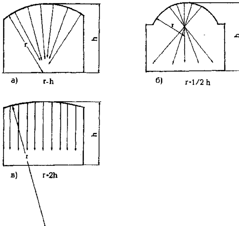
Рисунок 5 — Варианты решения зала с куполом
